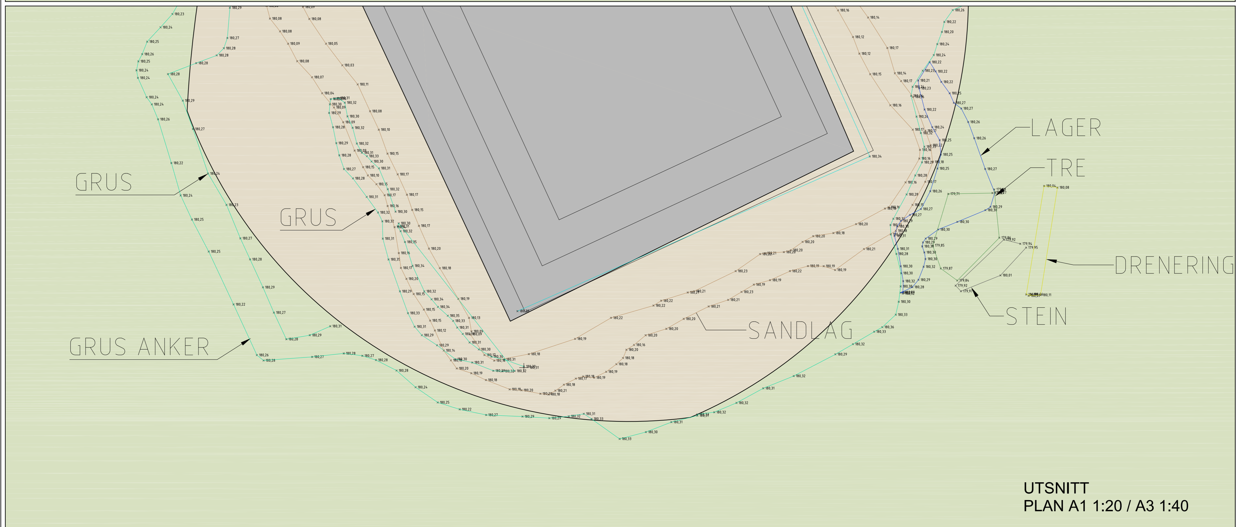
PLAN A1 1:50 / A3 1:100
